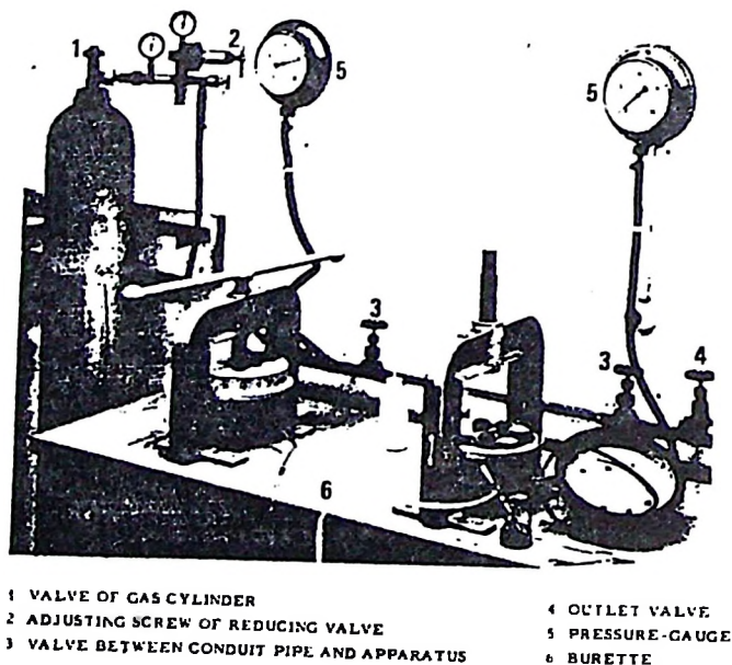
Fig. 13. Pressure membrane apparatus.
